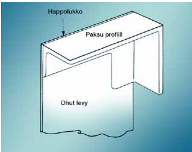
Kuva 7-7. Älä hitsaa yhteen kovin eri ainevahvuisia osia. Rakenne voi vetää sinkkiikylvyissä ja jäähdytyksessä eriaikaisen lämpenemisen ja jäähtymisen johdosta.
