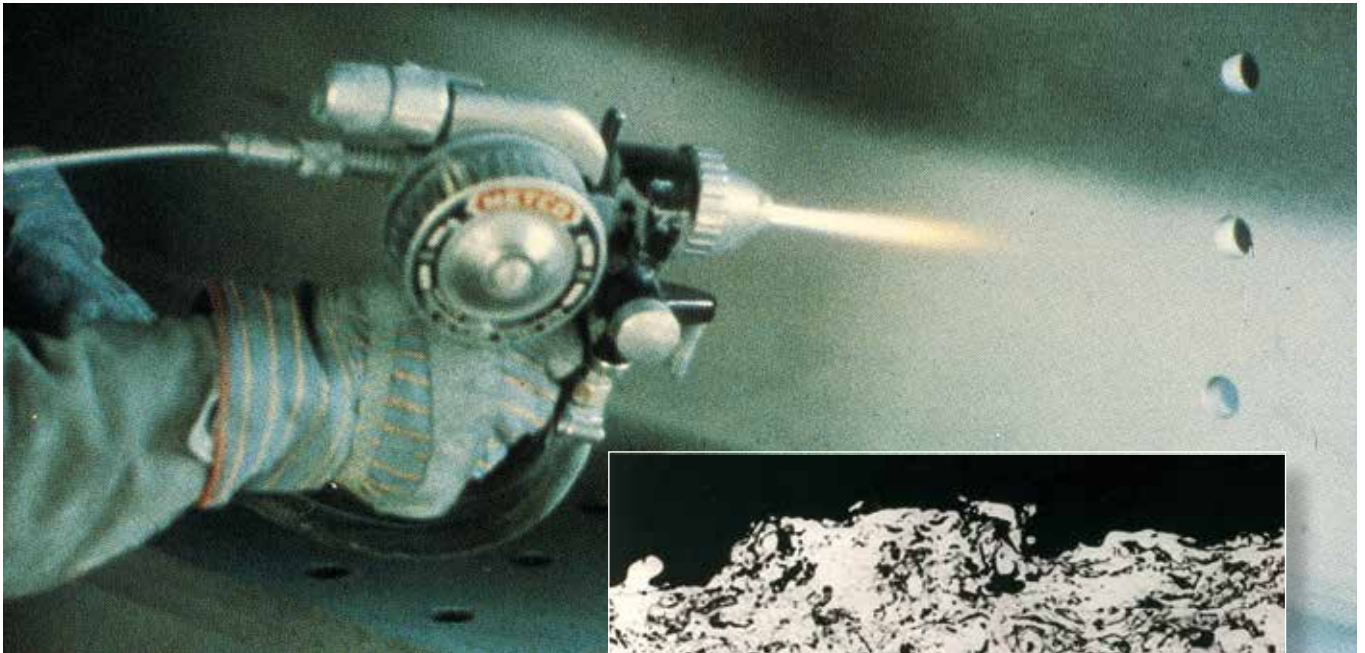
Kuva 3-2. Ruiskusinkitys.
