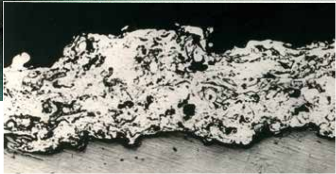
Kuva 3-3. Poikkileikkaus ruiskusinkitystä pinnoitteesta.
