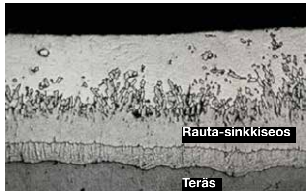
Kuva 5-2. Poikkileikkaus alumiinilla tiivistetyn teräksen sinkkipinnoitteesta.
