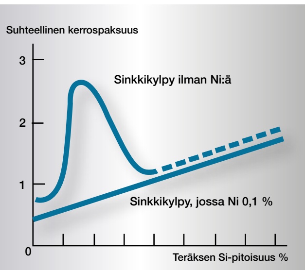
Kuva 5-8. Nikkelin lisääminen sinkkikylvyn vaikuttaa Sandelin-ilmiöön. Nikkeli ei enää vaikuta reaktiivisuuteen, kun teräksen piipitoisuus ylittää n. 0,22 % Si.
