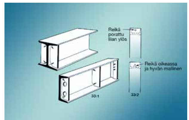
Kuva 7-12. Tukilevyjen kulmat on poistettava. Valumisaukot pitää sijoittaa niin lähelle pohjaa kuin mahdollista. Diagonaalien pää ei saa ulottua laippaan asti, tai sen pää on lovetettava. Huom. Vaihtoehto 2 muodostaa happopesäkkeen, jota pitää välttää.
