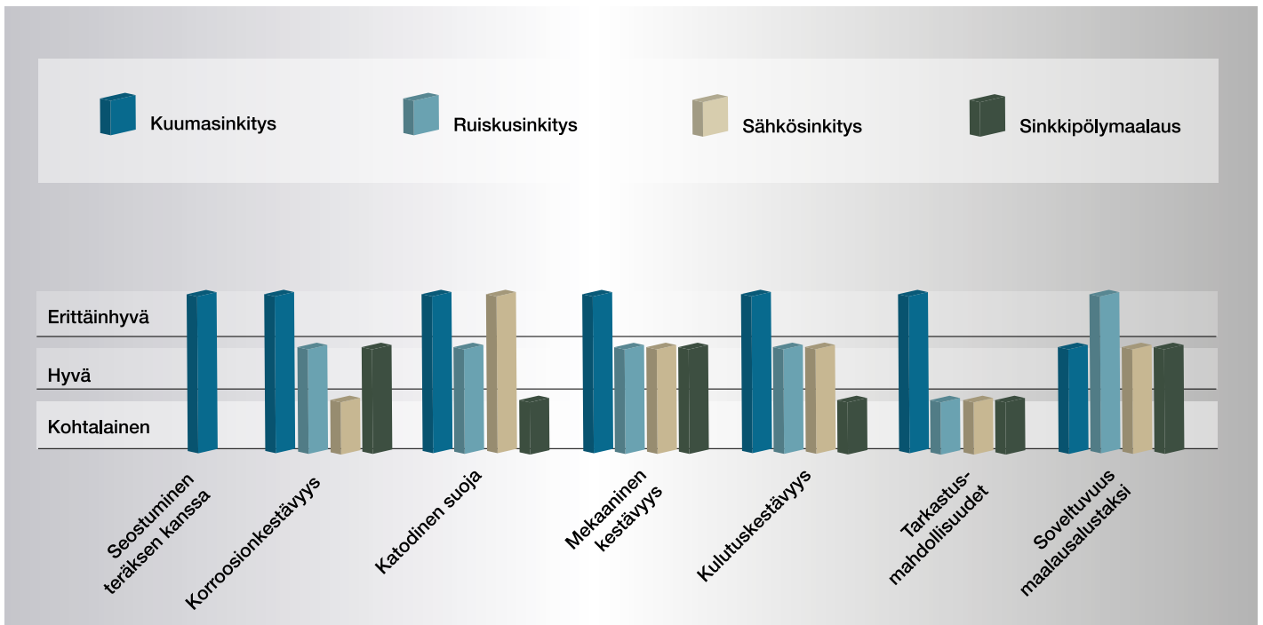
Kuva 3-5. Eri sinkkipinnoitteiden ja sinkkipölymaalain ominaisuuksien vertailu. Mekaaninen sinkitys ei ole mukana vertailussa, mutta sitä voidaan verrata lähinnä sähkösinkittyyn pinnoitteesen.
