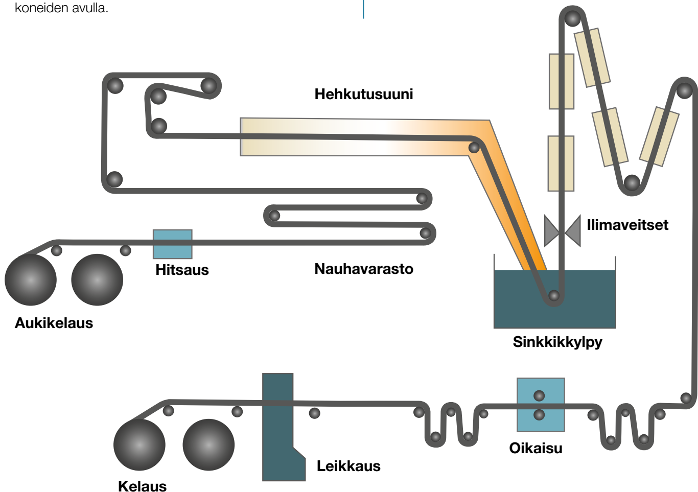
Kuva 4-8. Ohutlevyn jatkuvatoiminen kuumasinkitys.
