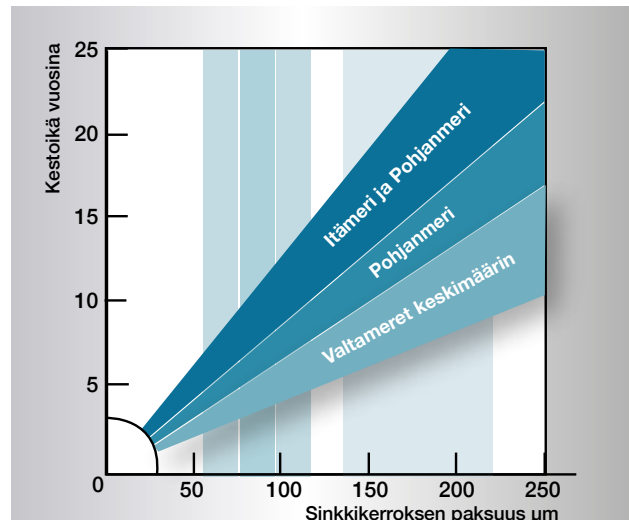
Kuva 10-3. Eripaksuisten sinkkikerrosten keskimääräinen kesto eri vesissä.
