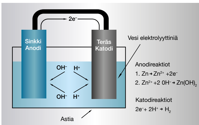
Kuva 10-8. Galvaaninen korrosio: sinkki kontaktissa teräkseen vedessä.
