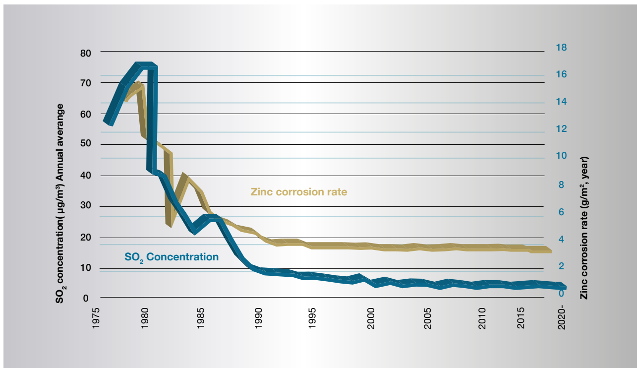
Kuva 1-1. Rikkidioksidipitoisuus ja sinkin syöpyminen Tuusulassa vuosina 1978 - 2020.
