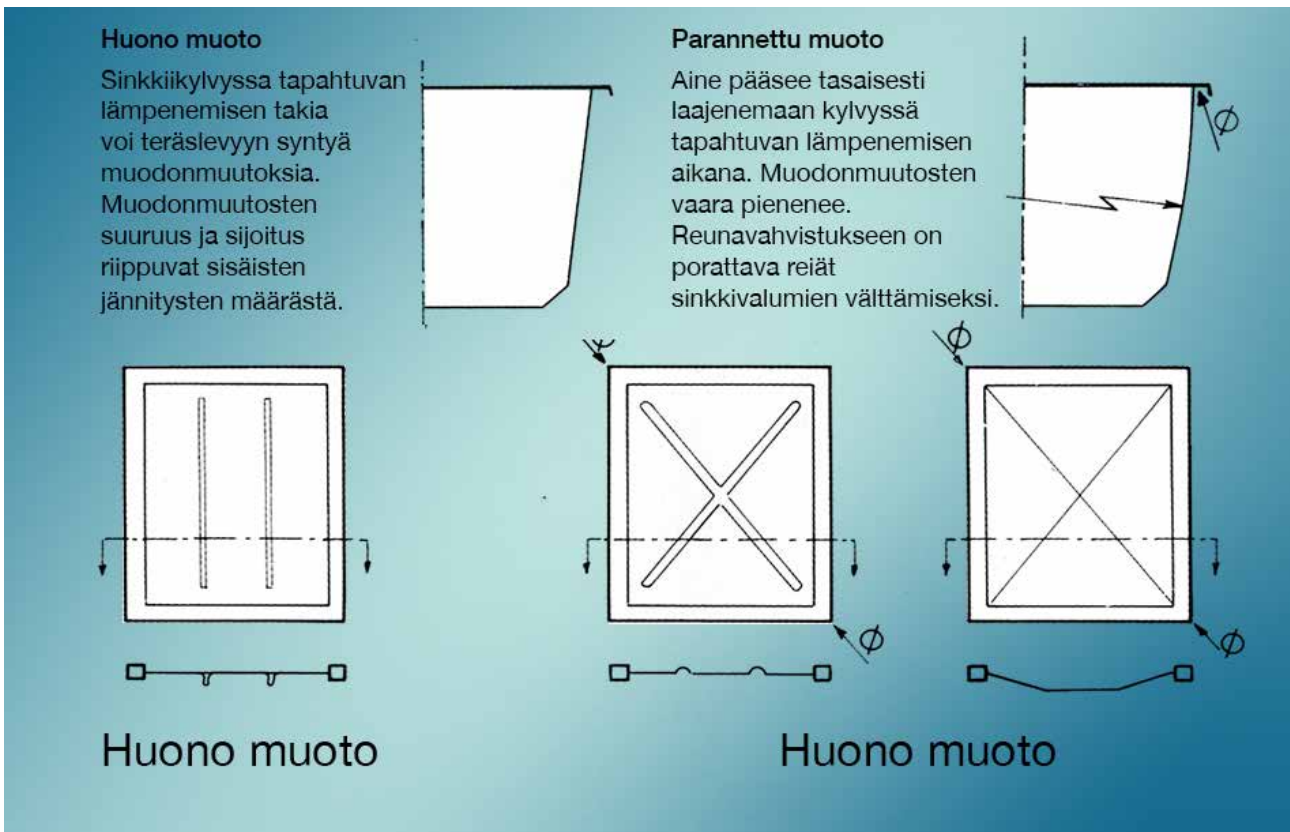
Kuva 7-9. Esimerkkejä jäykistämisestä tasopintojen muodonmuutosten pienentämiseksi.
