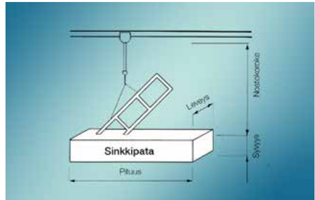
Kuva 7-2. Periaatekuva kuumasinkityksestä.
